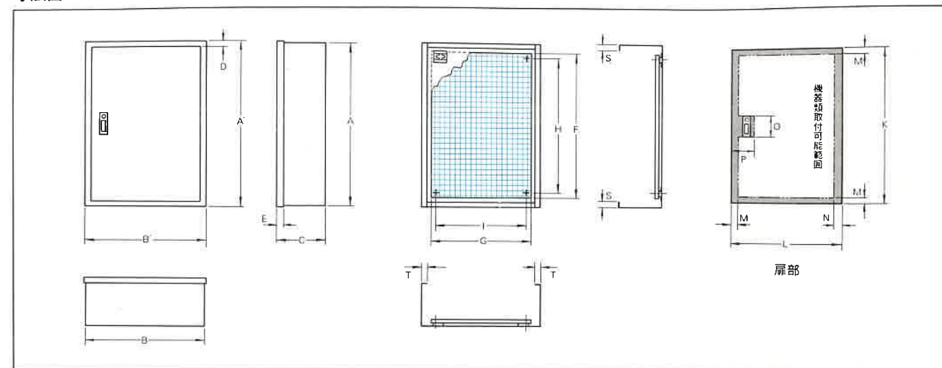
寸法図
