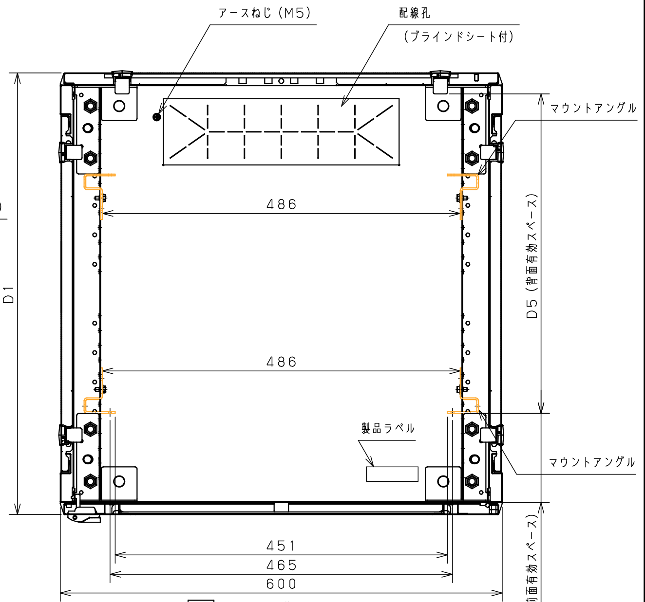
ヨコ断面
