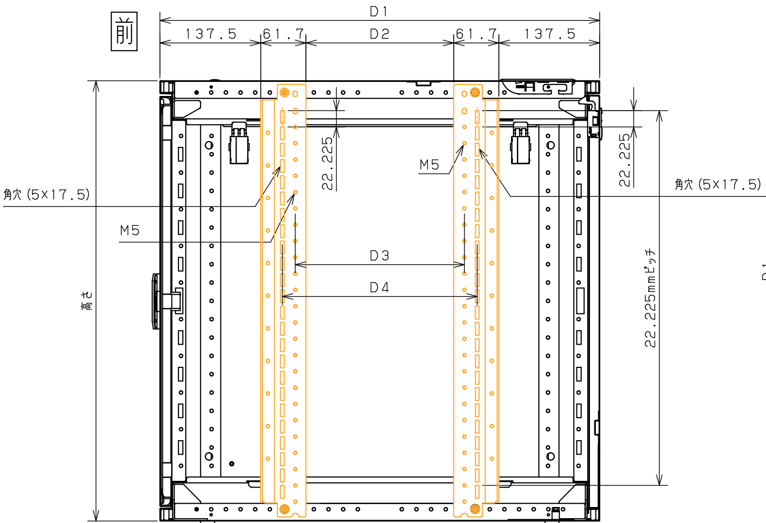
タテ断面
