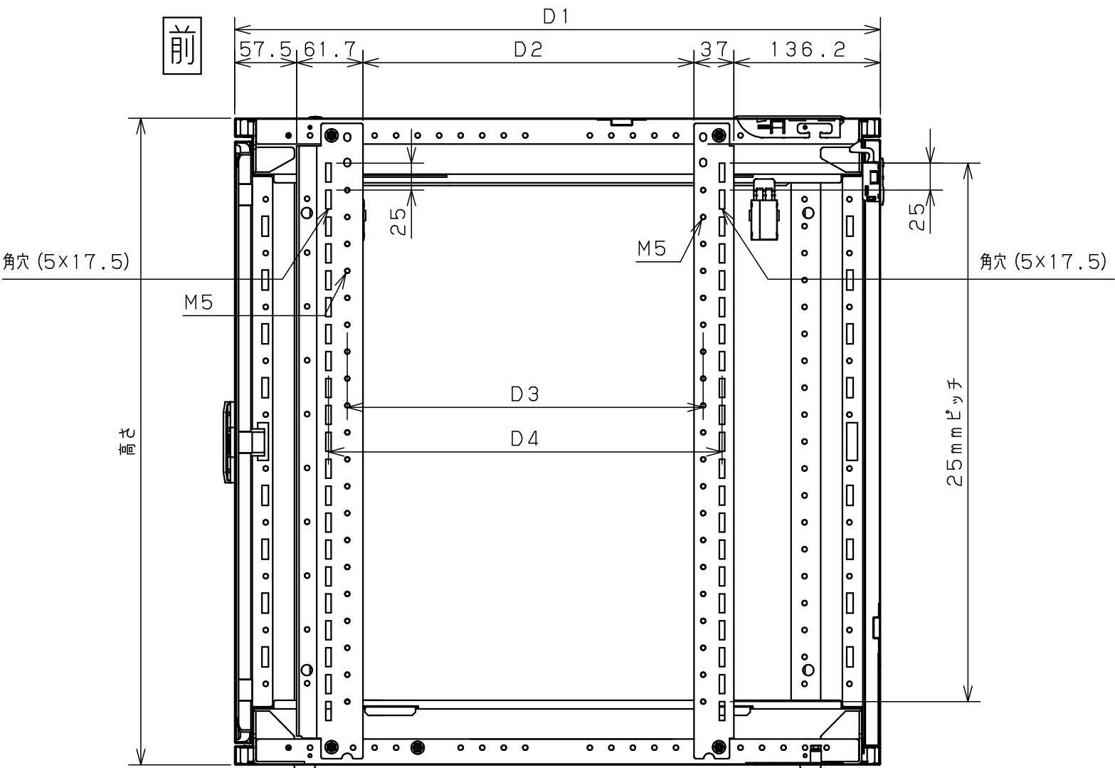
タテ断面
