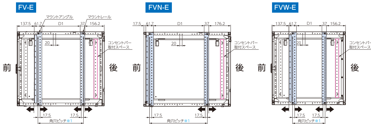
FV-E スタンダードタイプ
