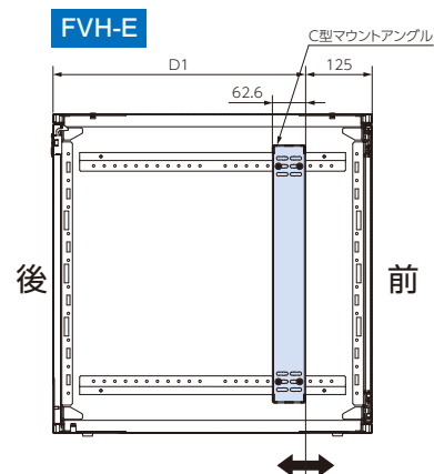
FVH-E HUB収納タイプ
