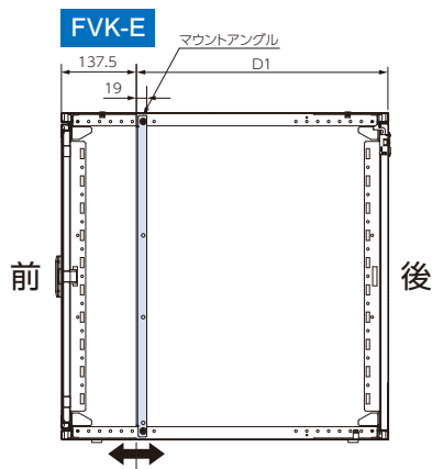
FVK-E 経済型スタンダードタイプ
