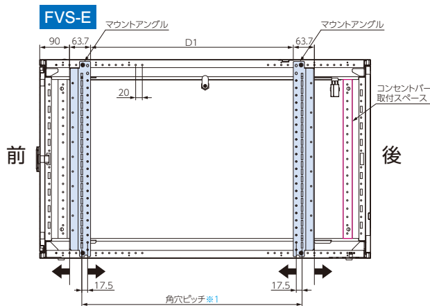
FVS-E サーバ収納タイプ
