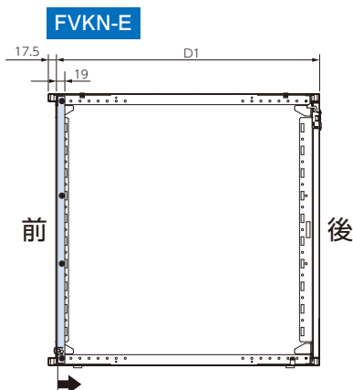
FVKN-E 経済型ドアなしタイプ
