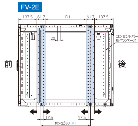
FV-2E (組替仕様) 前後マウントアングルタイプ
