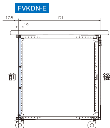
FVKDN-E ドアなしデスクタイプ
