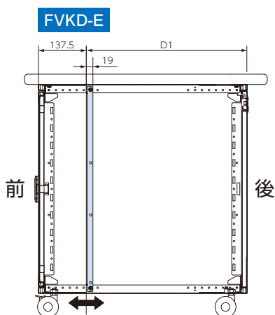
FVKD-E デスクタイプ
