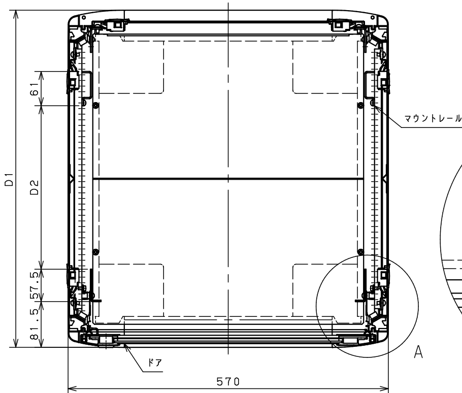
ドア付きタイプ (DARC)
