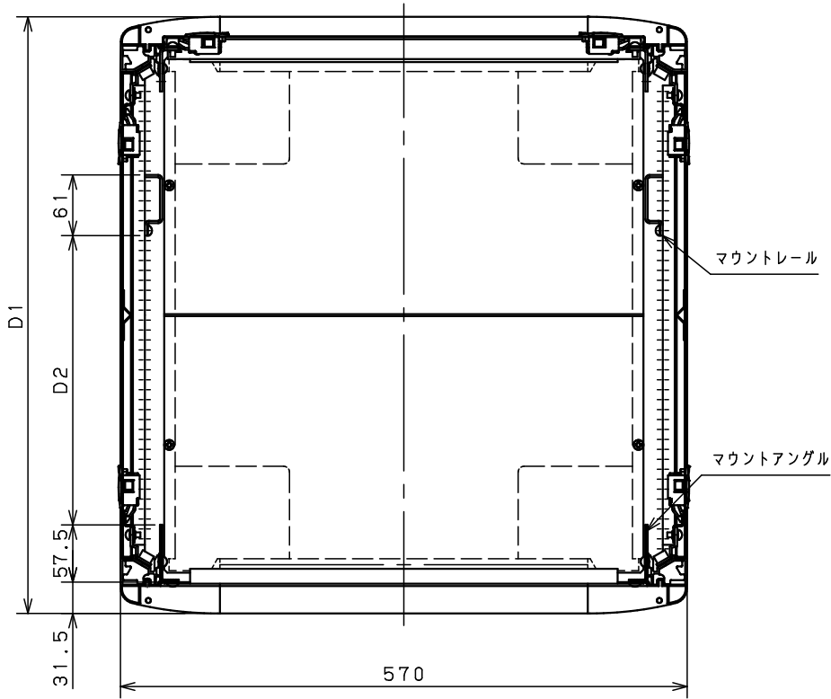
ドア無しタイプ (ARC)
