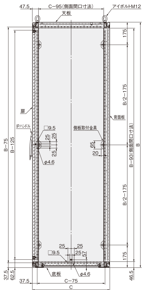
夕テ断面図
