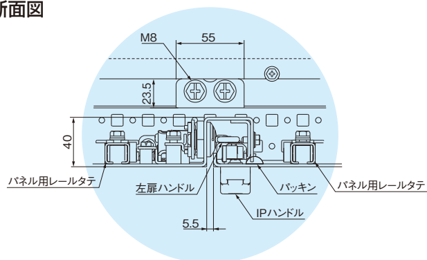
1 断面図
