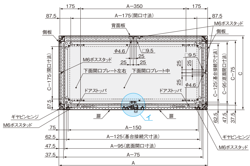
ヨコ断面図
